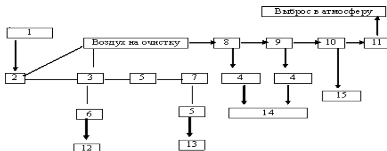
Рис. 2. Общая схема переработки ламп на установке «Экотром-2».
